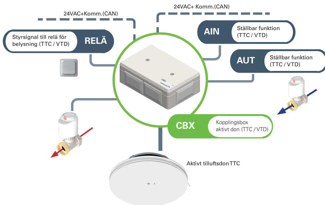
Anslutningsschema: Kopplingsbox CBX.
