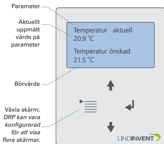
DRP i skärmvisningsläget "Tempkontroll"
