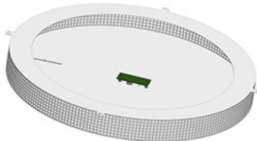
Säkerhetsgaller SHG Version D03 - vy från infästningssidan där ett kretskort för anslutning av rumstemperaturgivaren, närvarogivaren och IR finns tillgängliga för anslutning till det aktiva donet.
